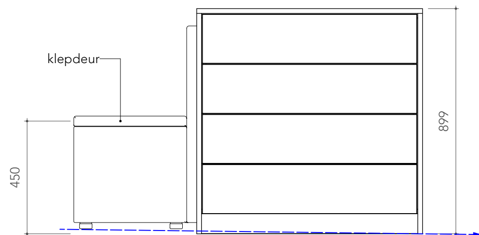
aanzicht raamzijde
